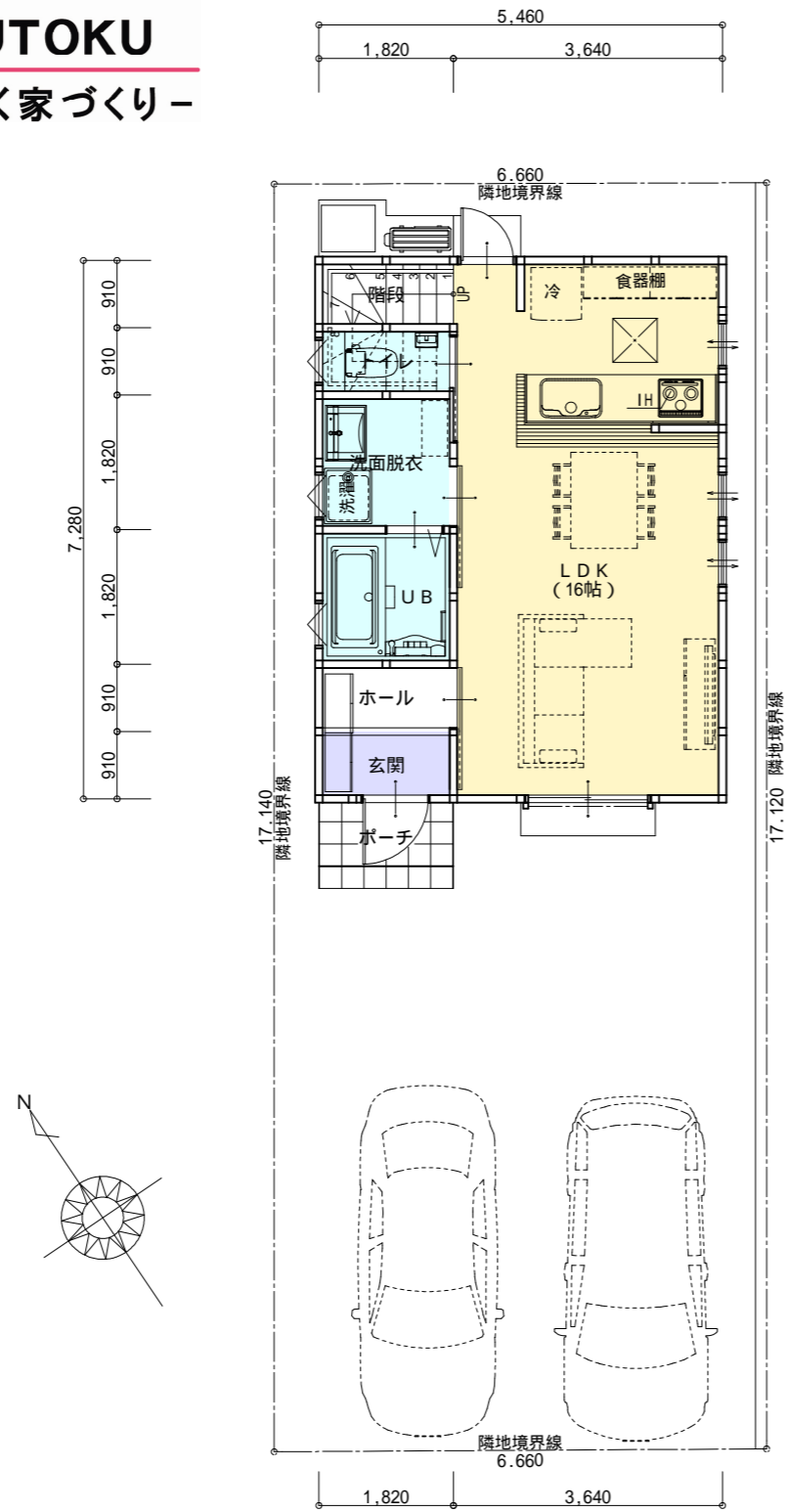
1階 平面図 S:1/100
