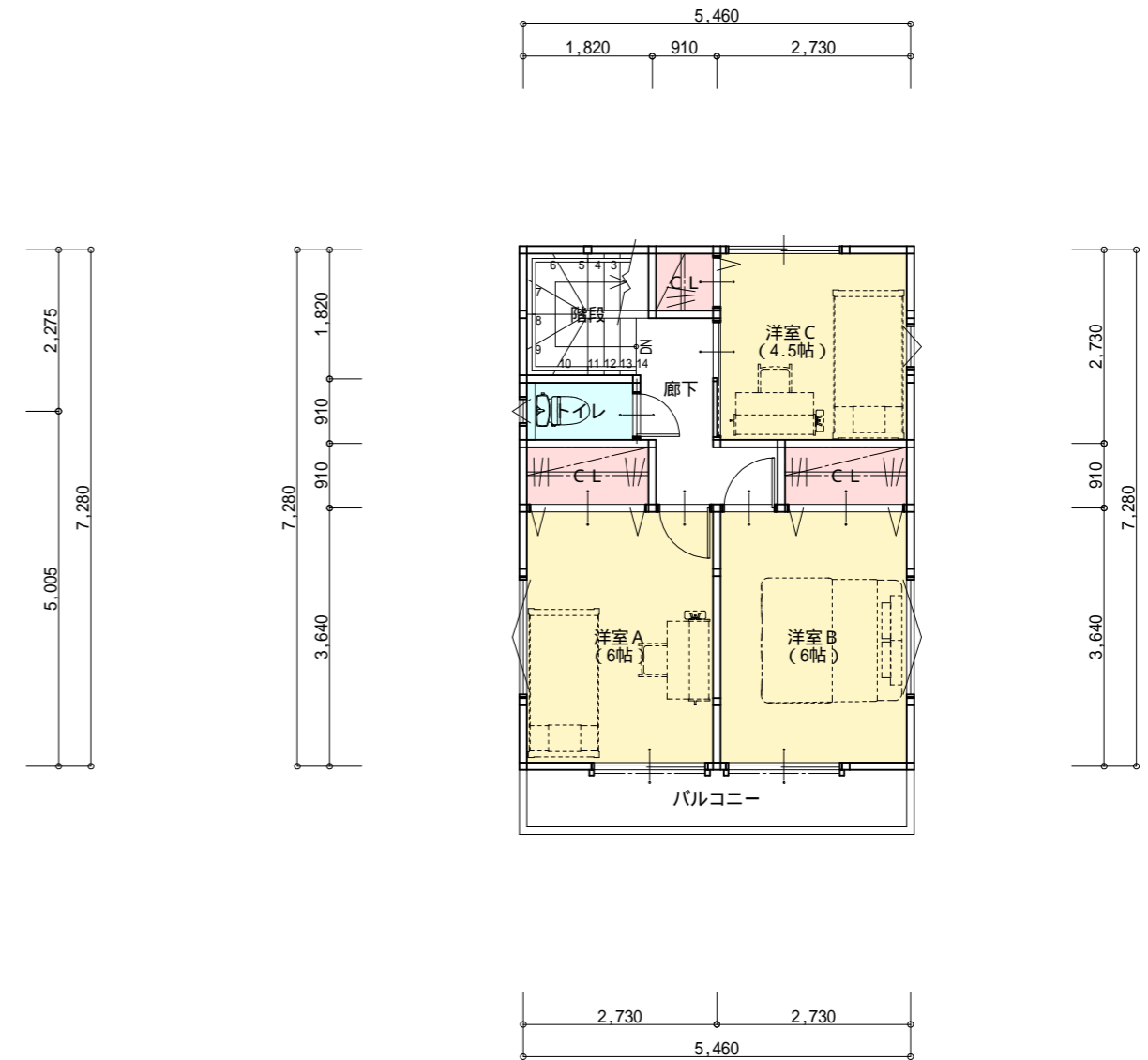
2階 平面図 S:1/100
